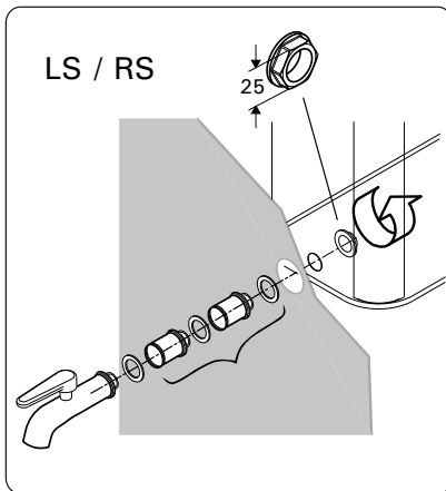
Vesihanan asennus. Montering av vattenkran.
