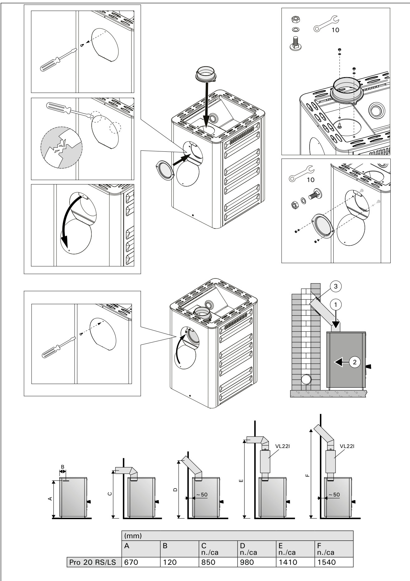
Obrázek 10. Připojení kamen ke zděři ve zdi z horního otvoru (všechny rozměry jsou uvedené v milimetrech)
