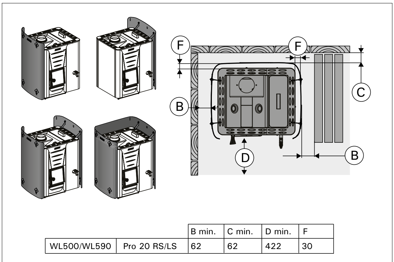
Figure 8. Distances de sécurité avec les gaines de protection (toutes les dimensions sont fournies en millimètres)
