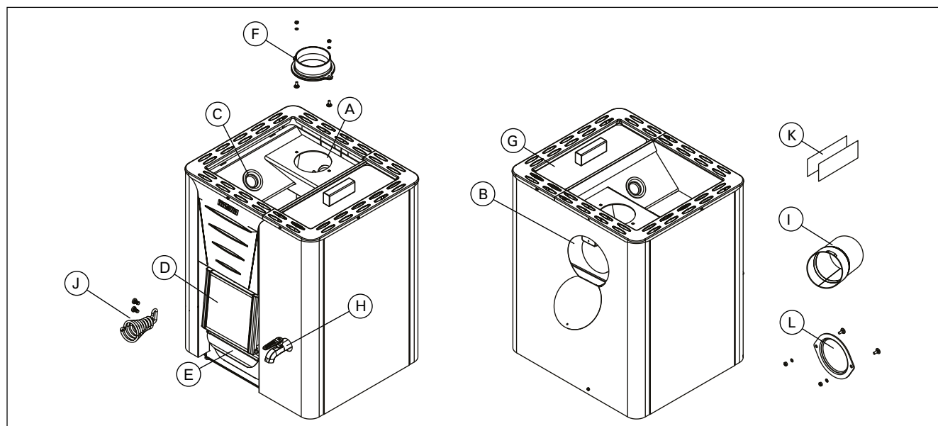
Obrázek 1. Součásti kamen. Neoprávněné úpravy kamen jsou zakázány. Figuur 1. Onderdelen van de kachel.
