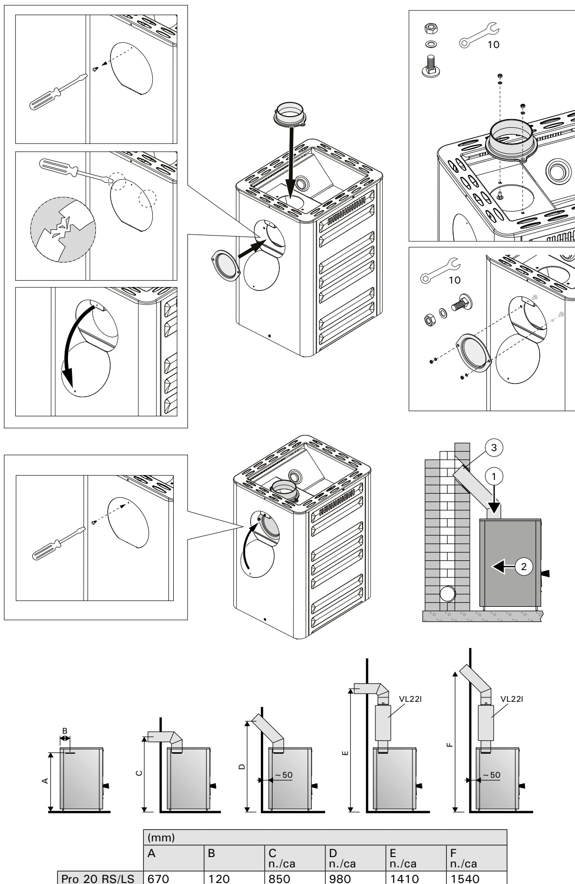
Figure 10. Raccordement du poêle à un conduit maçonné via l'ouverture de raccordement supérieure (toutes les dimensions sont fournies en millimètres)
