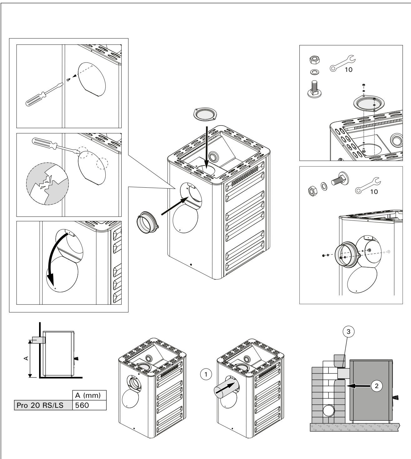
Kuva 9. Kiukaan liittäminen muurattuun savuhormiin takaliitäntäaukon kautta (mitat millimetreinä) Bild 9. Anslutning av ugnen till en murad röckkanal via den bakre anslutningsöppningen (måttan i millimeter)
